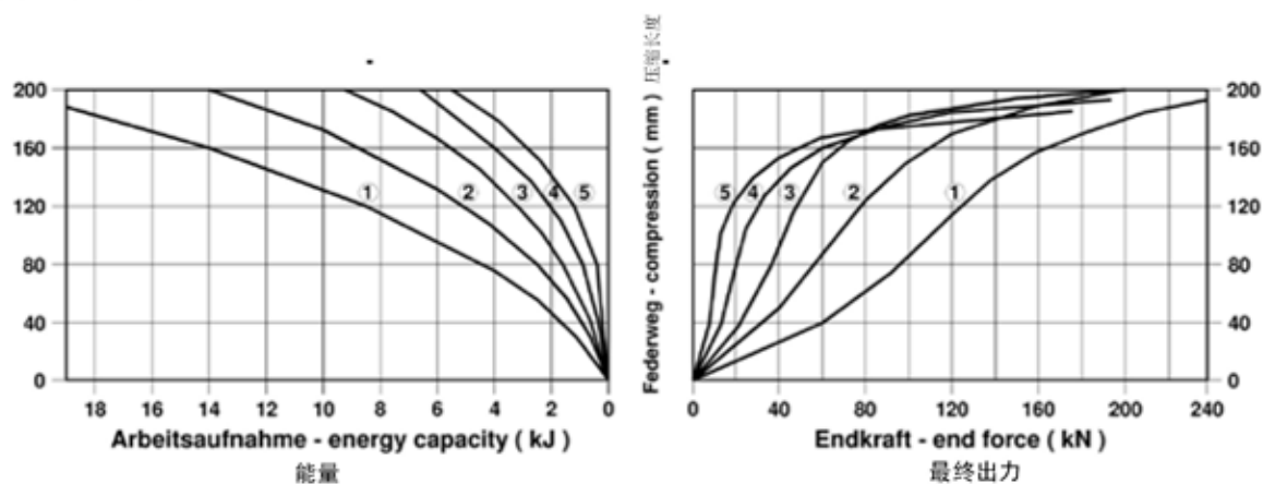
160 x 240蜂窝型聚氨酯缓冲器
