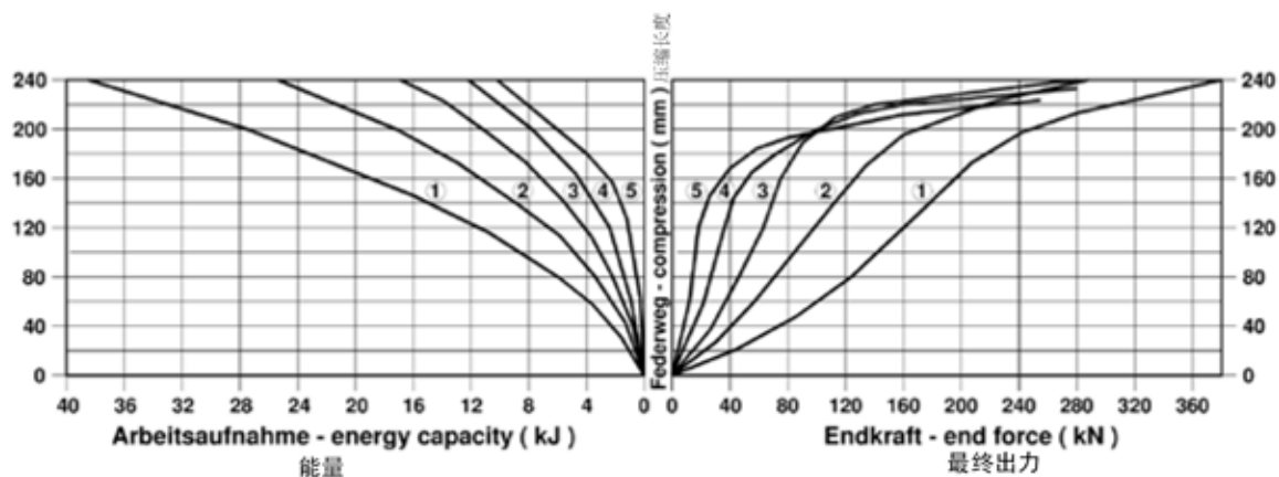
200 x 300蜂窝型聚氨酯缓冲器
