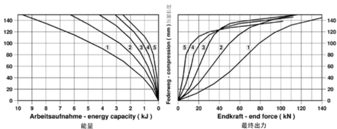
125 x 190蜂窝型聚氨酯缓冲器
