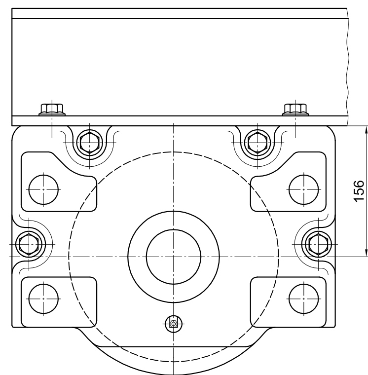
Plan de perçage de la construction annexe pour variante sur mesure
