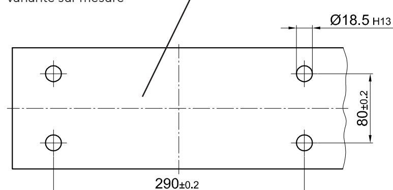
Plan de perçage de la construction annexe pour variante sur mesure
